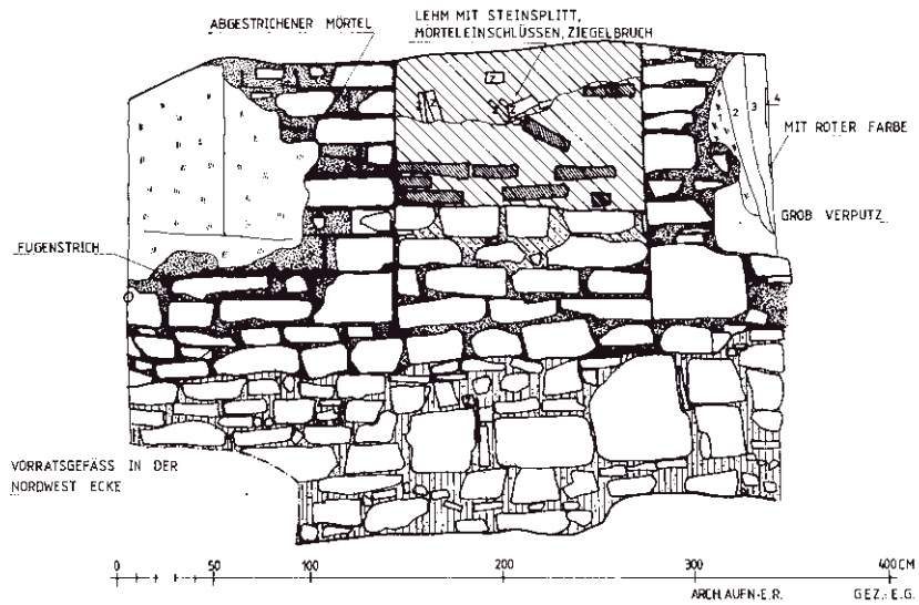
Abb. 47: 37, O-Mauer
