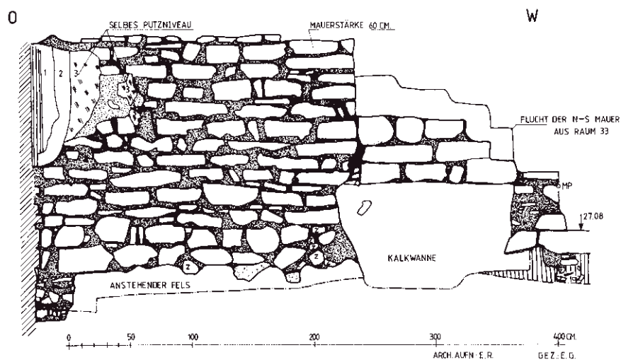
Abb. 48: 37, S-Mauer
